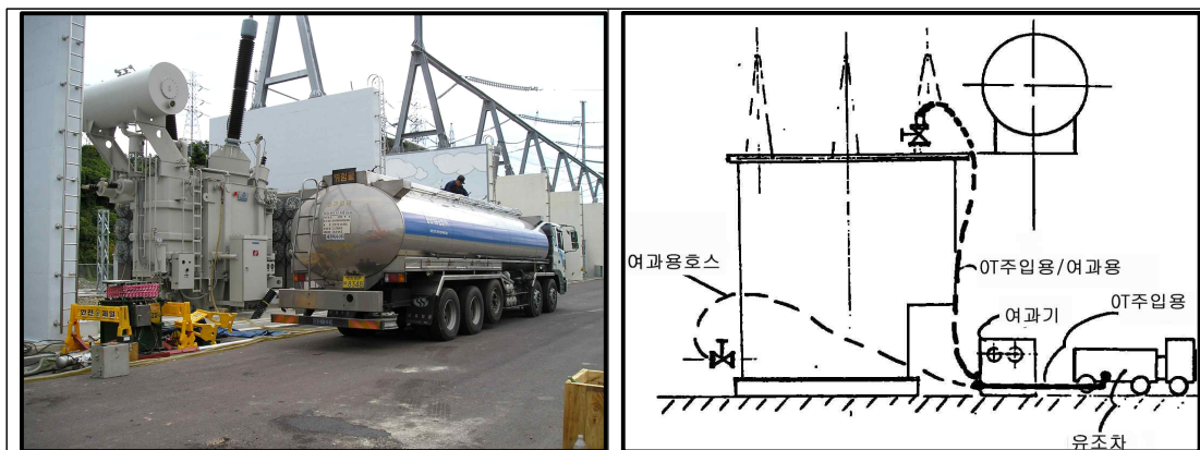
[그림] 주변압기 절연유 주유 및 여과
